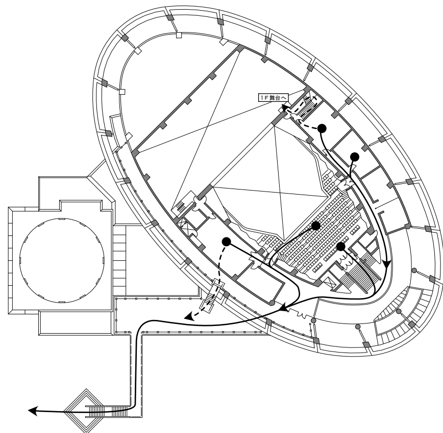
2階平面図
