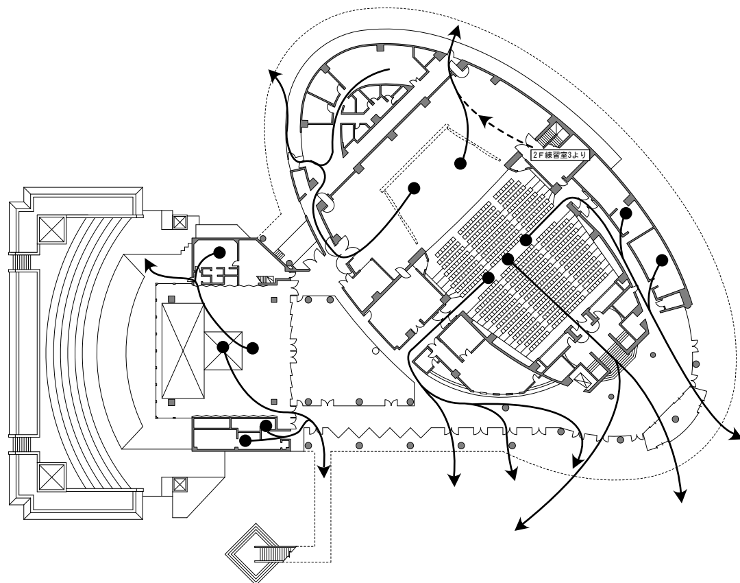
1階平面図
